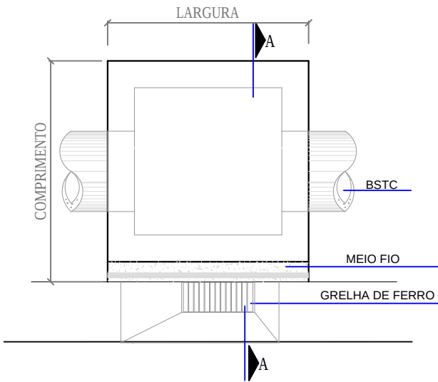
PLANTA BAIXA CAIXA DE CAPTAÇÃO
