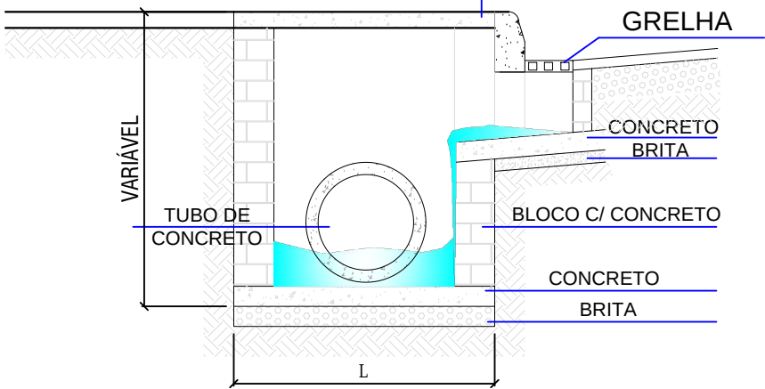
CAIXA DE CAPTAÇÃO CORTE A-A TAMPA CONCRETO
